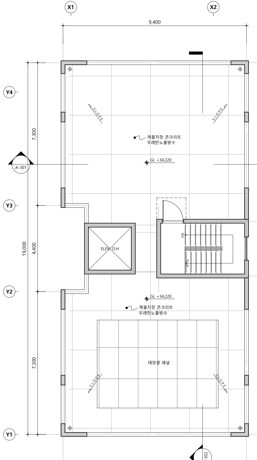
1 옥탑층 평면도 SCALE=1/100
